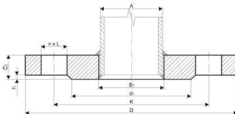
Plokščias flanšas, tipas O1 EN 1092-1:2001
